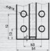
导轨横截与连接孔位尺寸
